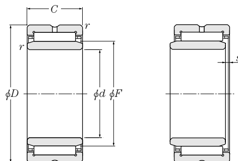
Type NA49 · R
