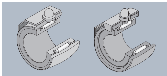
Fig. 1 Type FRIS · SA
