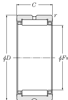
Type RNA49 · R ( F_w \geq 14\text{mm} ) Type RNA59 Type RNA69 · R Type NK · R ( F_w \geq 14\text{mm} )
